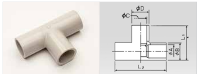
NDT-20, T-putki
