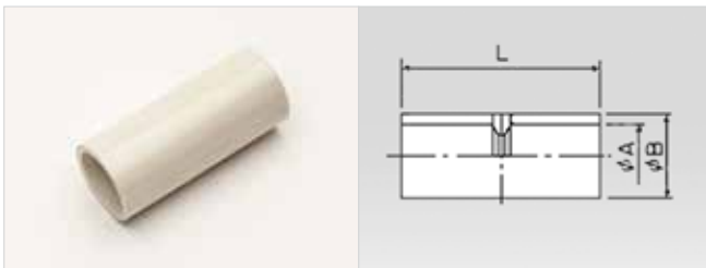
NDS-20, jatkos
